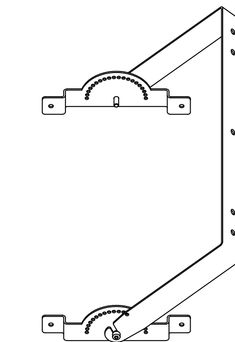
Кронштейн Mobile8CX
