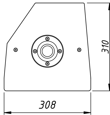
Вид Снизу
