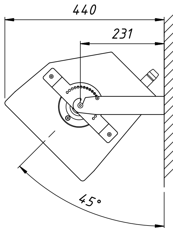
Крепление к стене
