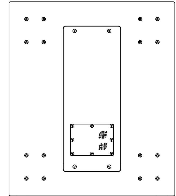
Вид Сзади
