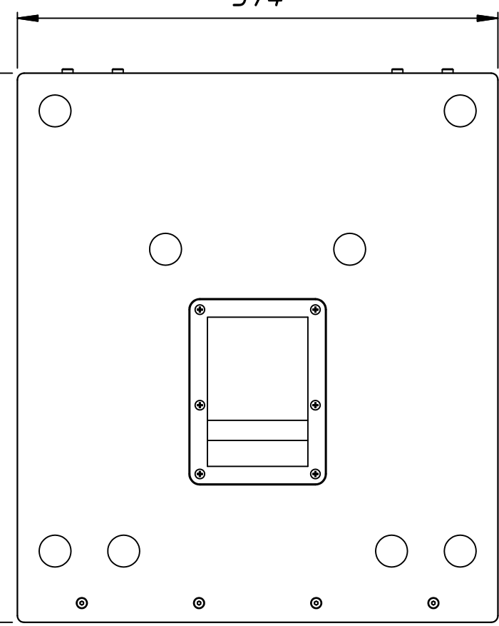
Вид Сверху
