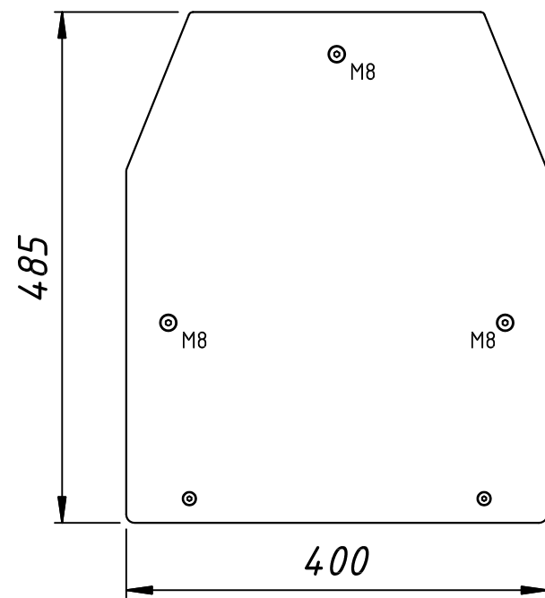
Вид Сверху
