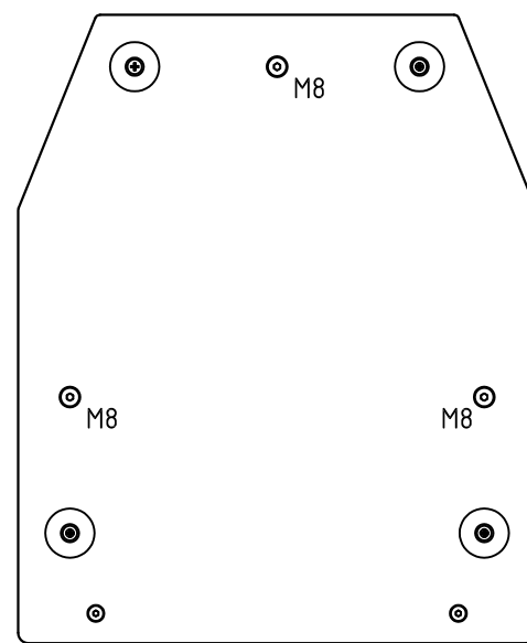
Вид Снизу
