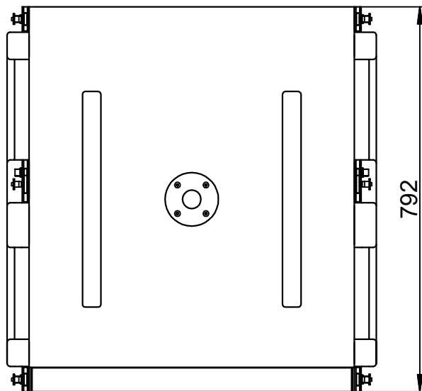
Вид сверху
