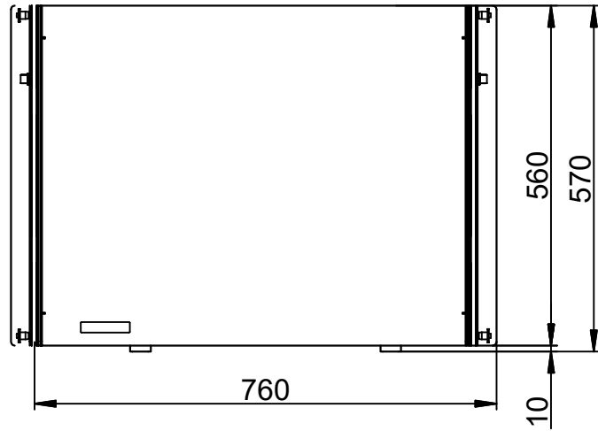
Вид спереди
