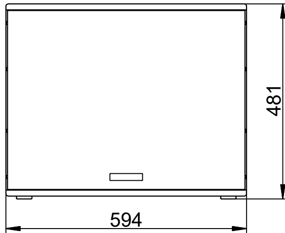
Вид спереди
